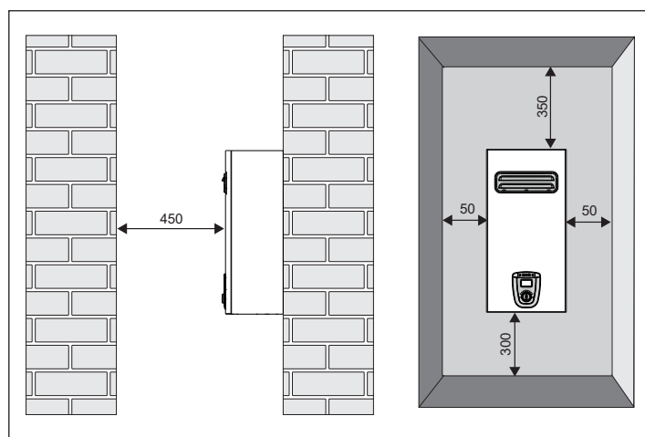
Fig. 7 - Distanze minime richieste per la manutenzione (in mm)
