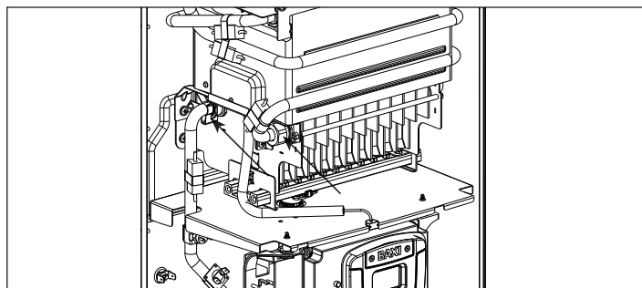
Fig. 29c - Smontaggio bruciatore
