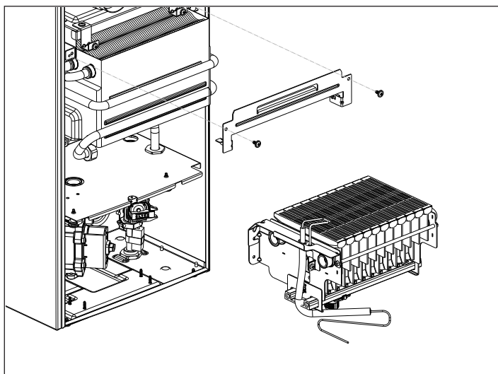
Fig. 30 - Smontaggio scambiatore
