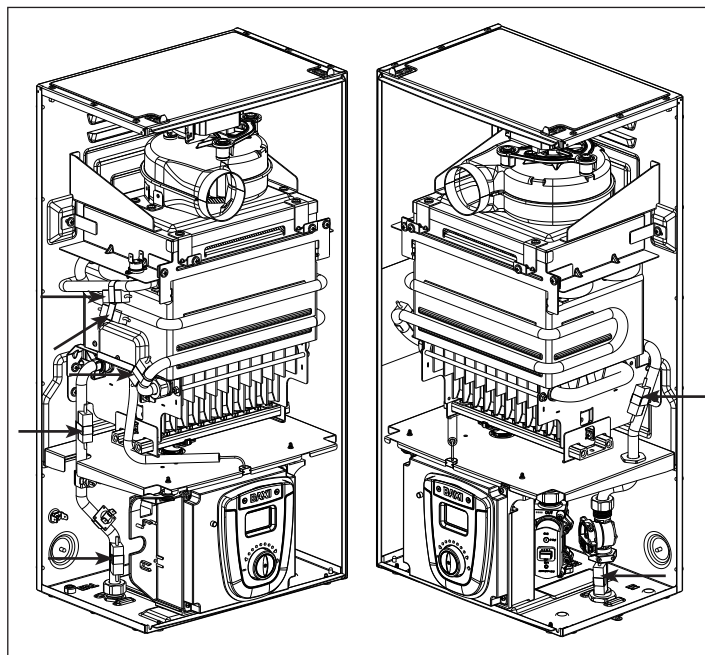
Fig. 10 - Posizionamento resistenze antigelo
