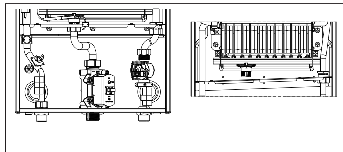
Fig. 14 - Smontaggio componenti
