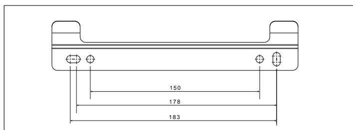
Fig. 8 - Staffa di sostegno
