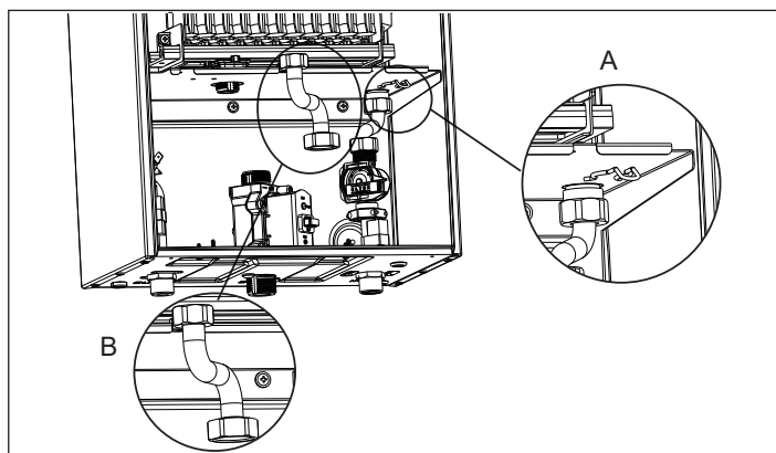
Fig. 29a - Smontaggio bruciatore
