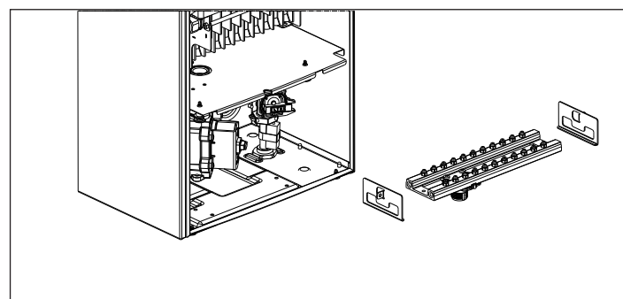
Fig. 15 - Smontaggio componenti
